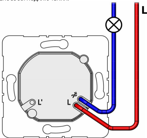
Типовое подключение диммера ISR-005-01 / DPI-01
